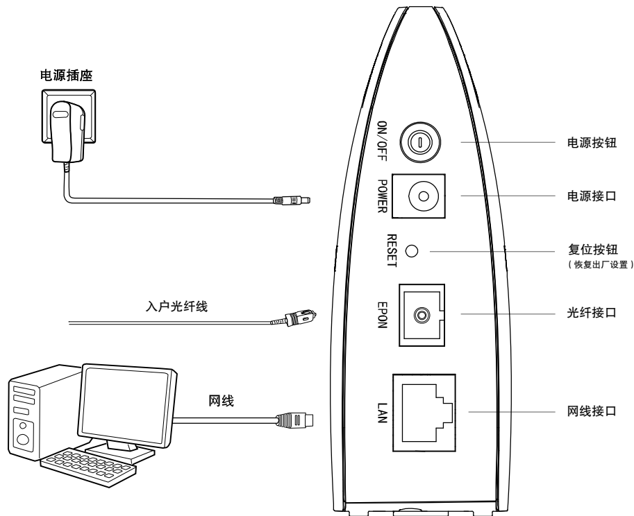
图 3-1 TL-EP112 硬件安装示意图
